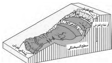
قسمت‌های اصلی یک زمین لغزش: ۱- ارتفاع لغزش، فاصله عمودی بین تاج لغزش تا پیشانی لغزش؛ ۲- سطح گسیختگی، سطح زیر بنا که توده لغزشی روی آن جابه‌جا می‌شود؛ ۳- تاج لغزش، بالاترین قسمت لغزش است.
