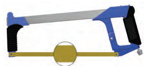
شکل ۱۱-۱ جهت دندان‌های اره
