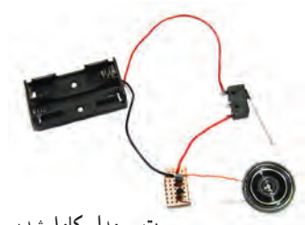
ت- مدار کامل شده
