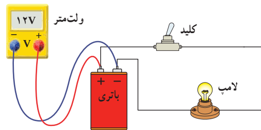
شکل ۱۶-۲ نحوه اتصال مولتی‌متر برای اندازه‌گیری ولتاژ
